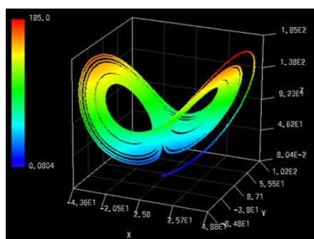
▲ローレンツ方程式の解曲線の計算と可視化
